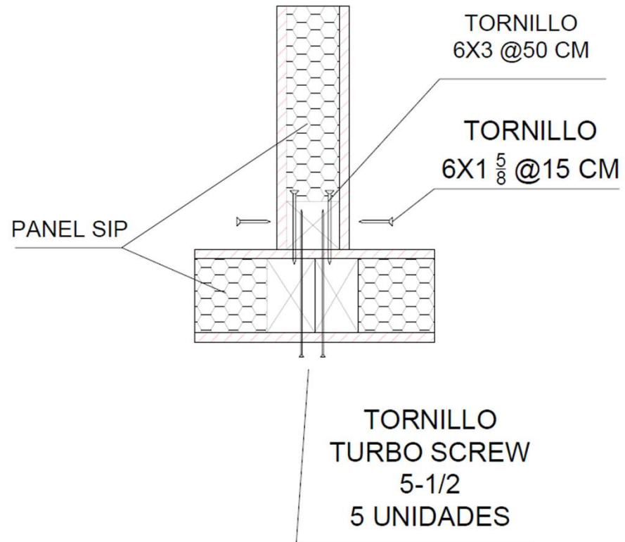
DETALLE TIPO 2 UNIÓN EN T
