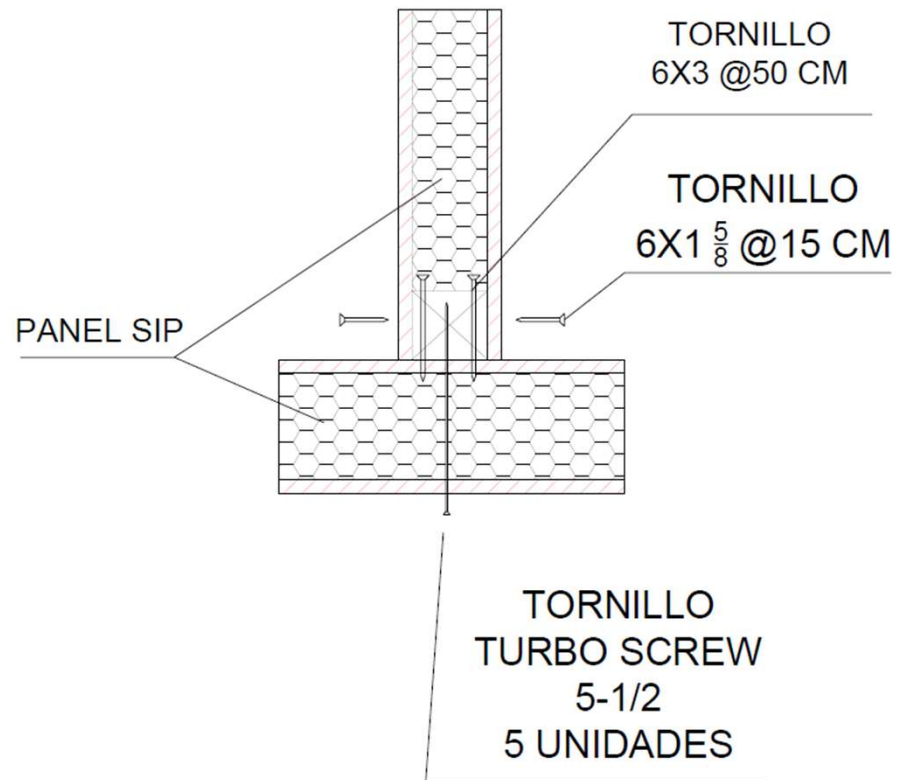
DETALLE TIPO 1 UNIÓN EN T
